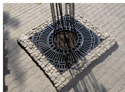
Krata żeliwna kwadratowa 125x125 cm / Φ50 cm KP-02
