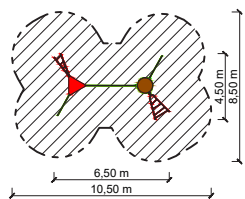
Elementy zestawu: wieża o rzucie trójkątnym oraz okrągłym, ścianka wspinaczkowa, drabinki, przeplotnia pajączyna
