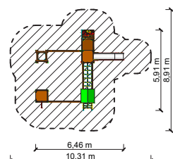
Elementy zestawu: wieża z daszkiem x1 i bez x3, wejścia: drabinka linowa, ścianka wspinaczkowa; mostek linowy, przeplotnia; zejścia: zjeżdżalnia.
