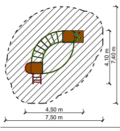
Elementy zestawu: wieża bez daszka x2, wejścia: drabinka; elementy sprawnościowe: drabinka dwustronna, przeplotnia, ścianka wspinaczkowa
