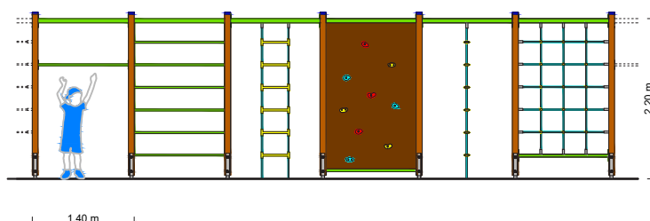
Zestaw zręcznościowy "Małpi gaj" - sześciokątny - 270x237x220 cm - stal lub drewno
