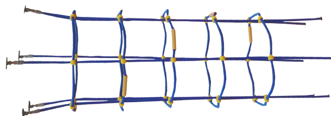
Siatka przejściowa/komin linowy
