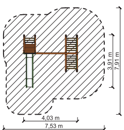
Elementy zestawu: podest, wejścia: drabinka; elementy sprawnościowe: drabinka dwustronna, przeplotnia; zejścia: zjeżdżalnia.
