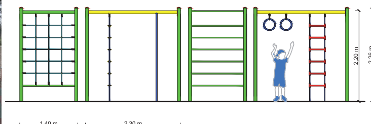
Zestaw zręcznościowy "Małpi gaj" - prostokątny - 230x140x220 cm - stal lub drewno
